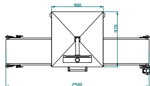
top view - vista dall'alto
